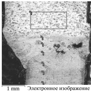
Рис. 9. Зоны определения химического состава образца: v = 450 мм/мин; \Delta F = -5 мм; \Delta t = -0,1 мм
