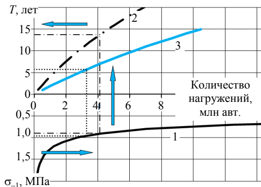
Рис. 2. Диаграмма определения прогнозируемых сроков усталостного разрушения дорожного покрытия с учетом вибрации: 1 – кривая усталости; 2 – то же виброн нагружения виброзащитного конструктивного варианта; 3 – то же традиционной конструкции
