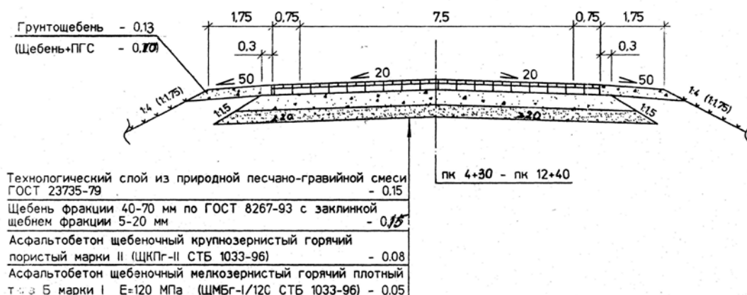
Рис. 1. Конструктивные элементы дорожной одежды
