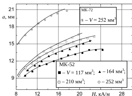
Рис. 5. Экспериментальная зависимость высоты a капель магнитных жидкостей разного объема V от напряженности магнитного поля H
