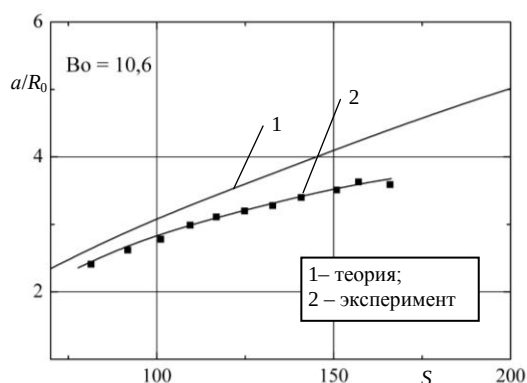
Рис. 7. Сравнение теоретической зависимости (5) относительной высоты a/R_0 капель магнитной жидкости от безразмерного магнитного критерия S при значении числа Бонда Bo = 10,6 с экспериментальными данными
