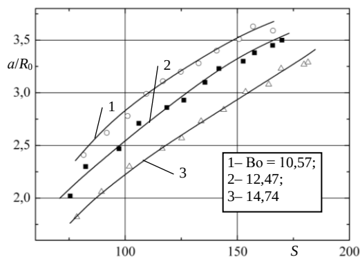
Рис. 6. Экспериментальная зависимость относительной высоты a/R_0 капель магнитной жидкости МК-52 от безразмерного магнитного критерия S при разных значениях числа Бо
