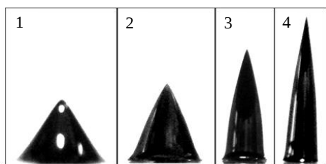
Рис. 4. Фотографии капель объемом V = 184 \text{ мм}^3 магнитных жидкостей M_s в магнитном поле с напряженностью H = 19,8 \text{ кА/м} с разной намагниченностью насыщения M_s (кА/м): 1 – 23,7; 2 – 34,2; 3 – 52,1; 4 – 72,5
