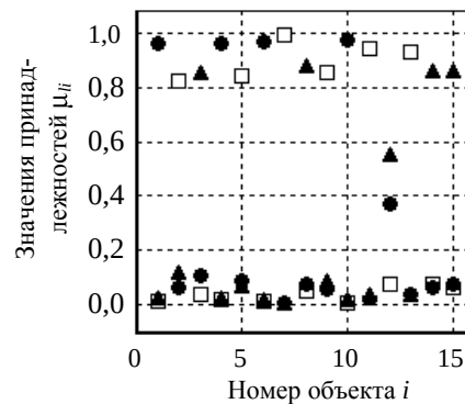
Рис. 5. Результат обработки множества объектов FCM-алгоритмом
