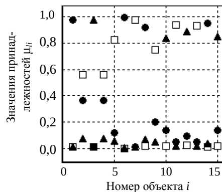
Рис. 6. Результат обработки множества объектов алгоритмом В. Педрича
