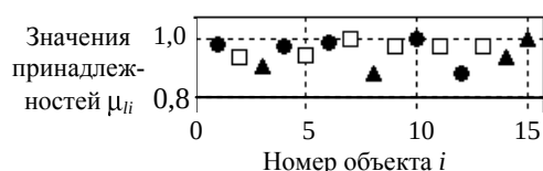
Рис. 2. Результат обработки множества объектов D-AFC(c)-алгоритмом
