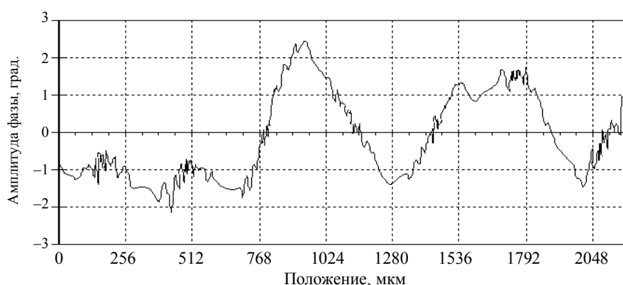
Рис. 6. График фазовой ошибки
