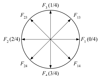
Рис. 4. Фазовая диаграмма сигналов датчика положения
