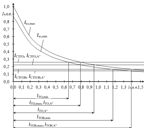
Рис. 1. Зоны мгновенного отключения микропроцессорной токовой защиты: l_{ТО,min} , l_{ТОВ,min} , l_{ТО,max} , l_{ТОВ,max} — зоны действия ТО и ТОВ для режимов двух- и трехфазного КЗ соответственно, если адаптивность защиты выведена; l_{ТО,A''} — зона действия первой ступени для первой конфигурации защиты; l_{ТО,A''} , l_{ТОВ,A''} — зоны действия ТО и ТОВ для второй конфигурации защиты; I_{CЗТО} , I_{CЗТОВ} , I_{CЗТО,A''} , I_{CЗТОВ,A''} — токи срабатывания первой и второй ступеней в случае выполнения защиты обычной и адаптивной (вторая конфигурация защиты) соответственно
