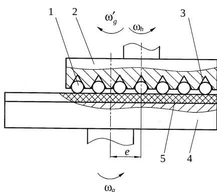
Рис. 1. Расположение дисков на начальном этапе шлифования
