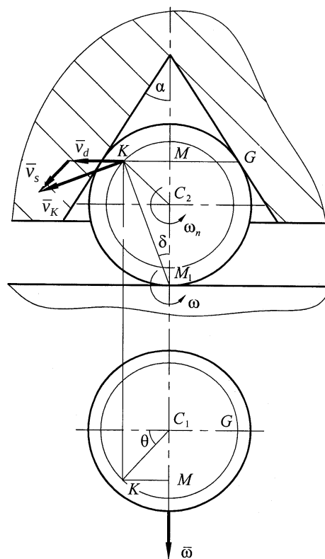
Рис. 3. К определению скорости скольжения шарика в коническом отверстии
