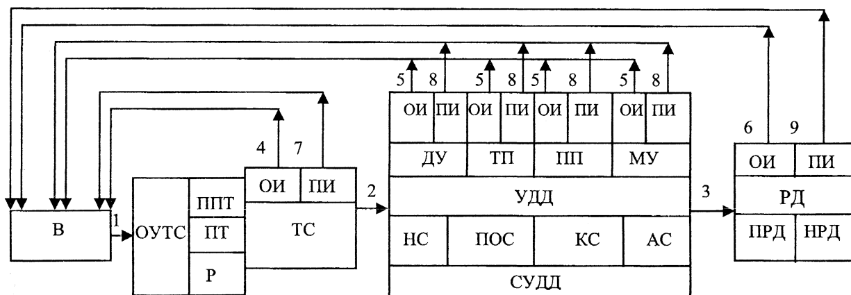
Рис. 2. Схема причинно-следственных связей между элементами сложной социально-детерминированной биомеханической системы «водитель – транспортное средство – условия дорожного движения», функционирующей по замкнутой схеме с обратной связью: В – водитель; ТС – транспортное средство; УДД – условия дорожного движения; РД – результат движения; ОУТС – органы управления транспортным средством; Р – руль; ПТ – педаль тормоза; ППТ – педаль подачи топлива; ДУ – дорожные условия; ТП – транспортный поток; ПП – пешеходный поток; МУ – метеорологические условия; СУДД – ситуации условий дорожного движения; НС – нормальная ситуация; ПОС – потенциально опасная ситуация; КС – конфликтная ситуация; АС – аварийная ситуация; ПРД – позитивный результат движения; НРД – негативный результат движения; ОИ – обстановка об информации об объекте наблюдения; ПИ – пусковая информация об объекте наблюдения; прямые причинно-следственные связи – 1, 2 и 3; обратные причинно-следственные связи – 4, 5, 6, 7, 8 и 9
