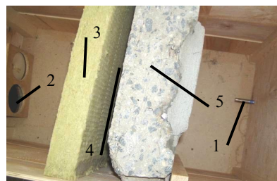
Рис. 4. 1 – микрофон шумомера; 2 – звуковые колонки; 3 – минераловатная плита; 4 – воздушная прослойка; 5 – бетонная стеновая панель
