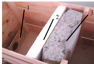
Рис. 3. 1 – звуковые колонки; 2 – плита пенополистирольная; 3 – бетонная стеновая панель
