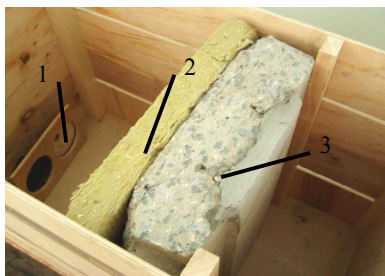
Рис. 2. 1 – звуковые колонки; 2 – минераловатная плита; 3 – бетонная стеновая панель
