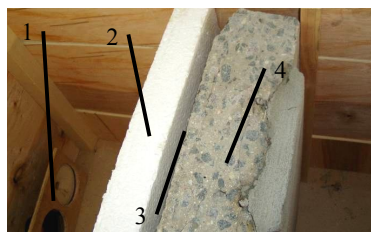
Рис. 5. 1 – звуковые колонки; 2 – пенополистирольная плита; 3 – воздушная прослойка; 4 – бетонная стеновая панель
