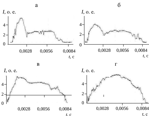
Рис. 3. Амплитуда и форма импульсов свечения плазмы в камере СВЧ плазмотрона при различных значениях величины емкости конденсатора в источнике питания: а – C = 0,5 мкФ; б – 1,0; в – 1,5; г – 2,0 мкФ
