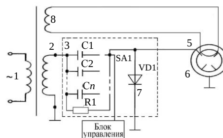
Рис. 1. Принципиальная электрическая схема высоковольтного источника питания СВЧ магнетрона
