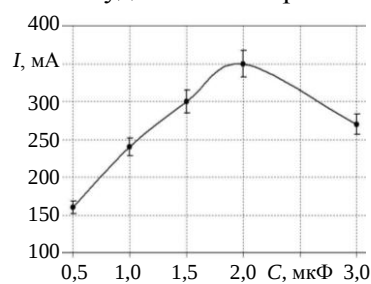
Рис. 2. Изменение величины выходного тока СВЧ магнетрона при изменении емкости в устройстве удвоения напряжения высоковольтного источника электропитания
