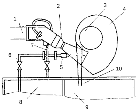
Рис. 5. Натрубный мокрый пылеулавливатель: 1 – дымоход; 2 – скруббер Вентури; 3 – дымоходная труба; 4 – улитка центробежного брызгоулавливателя; 5 – насосный агрегат шламочный; 6 – трубопровод всасывающий; 7 – трубопровод циркуляции воды; 8 – блок осветленного шлама; 9 – шламоулавливатель; 10 – рукав шламочный сливной
