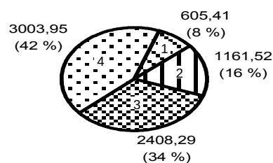
Рис. 3. Валовой объем выбросов загрязняющих веществ в атмосферу от асфальтосмесительных установок: 1 – SO 2 ; 2 – NO x ; 3 – CO; 4 – пыль неорганическая
