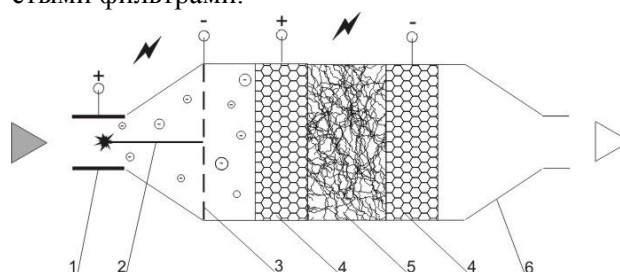
Рис. 1. Схема модели двухзонного аэрозольного электростатического фильтра: 1 – цилиндрический электрод; 2 – игольчатый коронирующий электрод; 3 – сетка-держатель коронирующего электрода; 4 – высокопористые проникаемые металлические электроды; 5 – фильтрующий полимерный материал; 6 – корпус
