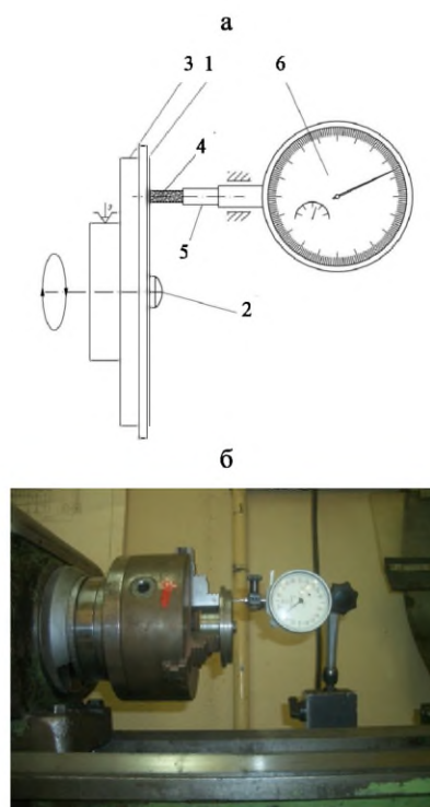
Рис. 4. Установка для оценки абразивной способности и износостойкости алмазосодержащего покрытия на боковых поверхностях распиловочных дисков: а – принципиальная схема; б – общий вид экспериментальной установки; 1 – распиловочный диск; 2 – центральный болт; 3 – планшайба; 4 – истираемый образец; 5 – измерительный шток индикатора; 6 – индикатор МИГ-1
