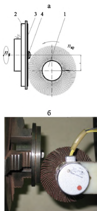
Рис. 3. Обработка боковых поверхностей распиловочного диска абразивным лепестковым кругом: а – технологическая схема обработки; б – общий вид экспериментальной установки; 1 – лепестковый круг; 2 – планшайба; 3 – распиловочный диск; 4 – зажимной винт
