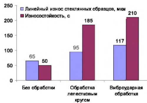
Рис. 5. Значения линейного износа стеклянных образцов и износостойкости алмазосодержащего покрытия, полученного на поверхности испытуемых распиловочных дисков
