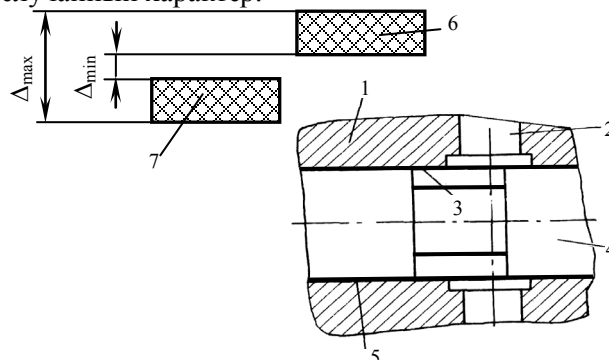
Рис. 3. Гидрораспределитель
