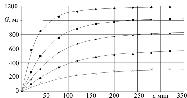
Рис. 4. Зависимость G = f(C_{исх}, t) при распаде дисперсных систем с различной высотой слоя эмульсии h : точки – опыт; линии – расчет; \diamond – h = 100 см; \blacksquare – 80; \blacktriangle – 60; \bullet – 40; \times – 20 см
