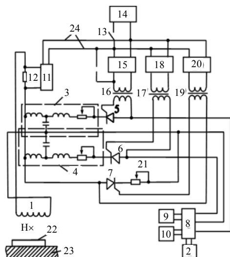
Рис. 1. Схема экспериментальной установки для исследования распространения импульсных магнитных полей: 1 – излучатель импульсного магнитного поля; 2 – источник питания; 3, 4 – формирующие линии; 5, 6, 7 – тиристоры; 8 – блок управления; 9, 10 – накопительные конденсаторы; 11 – измерительный прибор; 12 – измерительное сопротивление; 13 – электрический ключ; 14 – источник постоянного напряжения; 15 – электронная схема; 16, 17 – трансформаторы запуска тиристоров; 18 – электронная схема; 19 – трансформатор запуска тиристора; 20 – электронная схема; 21 – потенциометр; 22 – датчик магнитного поля; 23 – металлический образец; 24 – линия синхронизации
