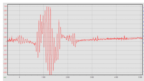
Рис. 6. Зависимость величины электрического напряжения, снимаемого с индукционной магнитной головки, от времени (пластина из алюминия толщиной 3 \cdot 10^{-5} м)
