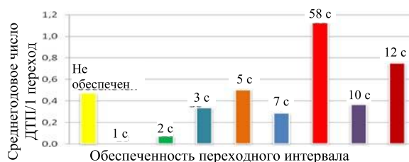
Рис. 8. Влияние отсутствия индикатора обратного отсчета при обеспеченности переходного интервала
