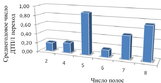
Рис. 1. Влияние количества полос на безопасность движения пешеходов
