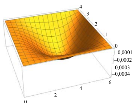
Рис. 2. Поверхность прогибов плиты
