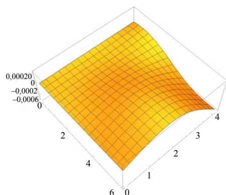
Рис. 4. Поверхность прогибов в прямоугольной плите с двумя опорными краями
