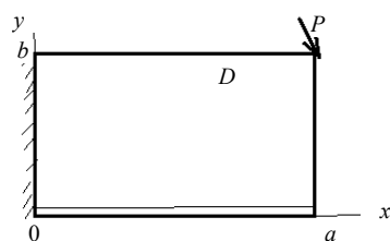
Рис. 3. Прямоугольная плита, нагруженная угловой силой
