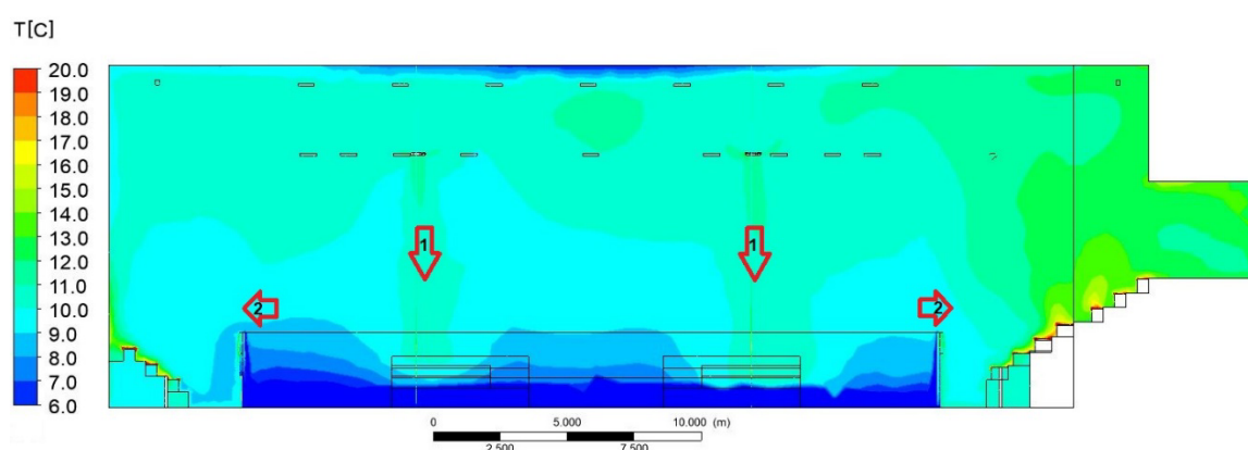
Рис. 3. Распределение температуры во внутреннем пространстве ледовой арены:
