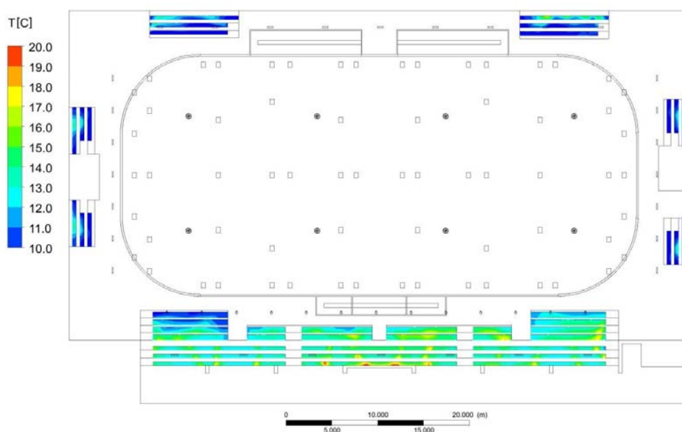
Рис. 2. Распределение температуры в зоне расположения зрителей на трибунах
