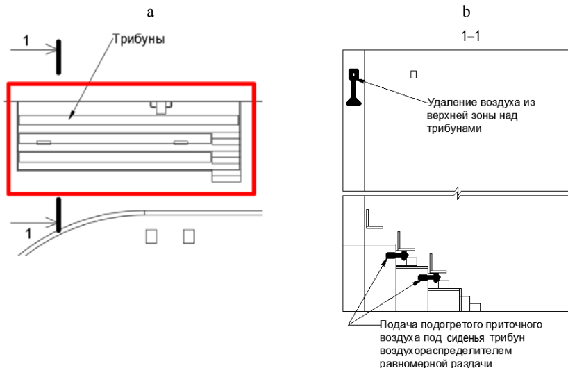
Рис. 4. Фрагмент плана (а) с размещением трибуны для зрителей и разрез 1–1 (b) с размещением приточных воздухораспределителей и вытяжных решеток (техническое решение 1)
