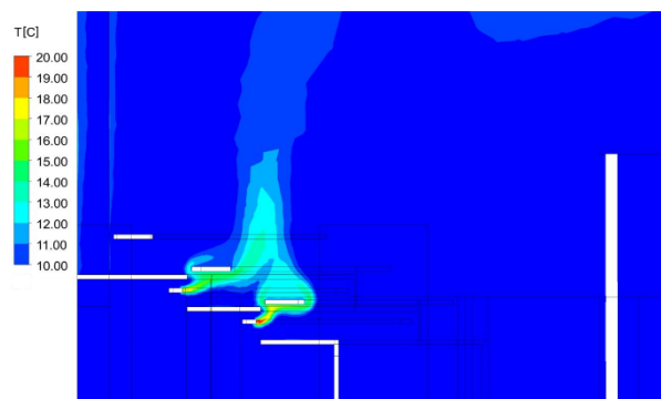
Рис. 5. Распределение температуры по разрезу 1–1 трибуны для зрителей
