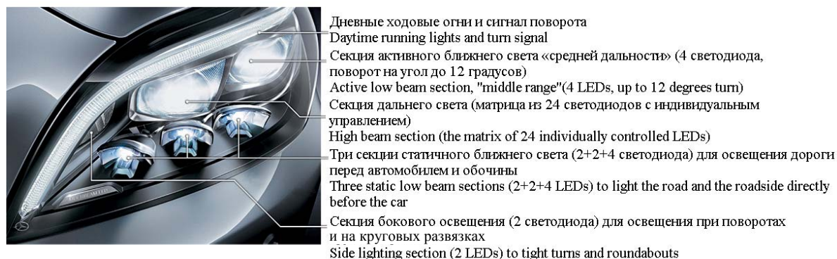
Рис. 6. Фара Multibeam автомобиля Mercedes CLS 500
