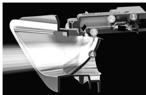
Рис. 1. Конструкция лазерной фары серийного гибридного автомобиля BMW i8 [3]: 1 – лазерные диоды; 2 – оптическая система; 3 – пластина с люминофором; 4 – металлический рефлектор
