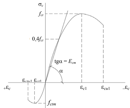
Рис. 3. Зависимость «напряжение – относительная деформация» для бетона: \epsilon_c – относительная деформация бетона; \epsilon_{c1} – то же, соответствующая прочности бетона на сжатие; \epsilon_{cul} , \epsilon_{ctu1} – то же, соответствующая предельному сжатию и растяжению бетона; \epsilon_{ctl} – то же, соответствующая прочности бетона на растяжение; f_{cm} – средняя прочность на осевое сжатие бетона нормального веса; f_{ctm} – то же на осевое растяжение бетона нормального веса, установленная для проектирования конструкций; E_{cm} – модуль упругости бетона; \sigma_c – нормальное напряжение в бетоне
