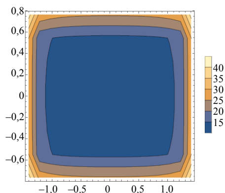
Рис. 6. Изополя давлений под плитой (кПа) при центральном нагружении силой F = 100 кН
