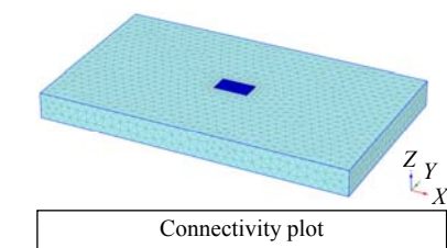
Рис. 10. Сетка конечных элементов
