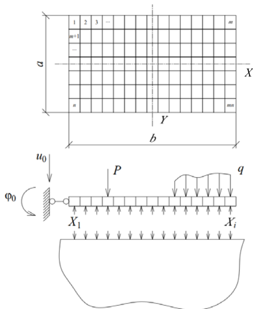
Рис. 1. Основная система способа Жемочкина: u_0, \varphi_0 – линейное и угловое перемещения введенного заземления на плите; P, q – произвольные сосредоточенная и распределенная нагрузки; X_1, X_i – усилие в связи 1-го и i -го участков Жемочкина
