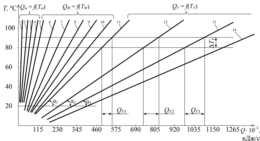
Рис. 2. Зависимость температуры теплоносителей от количества подведенной теплоты: 1 – расход масла V_M = 10 л/мин; 2 – 20; 3 – 30; 4 – 40 л/мин; 5 – расход воздушного теплоносителя W = 4000 м³/ч; 6 – 6000; 7 – 8000; 8 – 10000; 9 – 12000; 10 – 14000 м³/ч; 11 – расход жидкостного теплоносителя V = 80 л/мин; 12 – 120; 13 – 160; 14 – 200 л/мин
