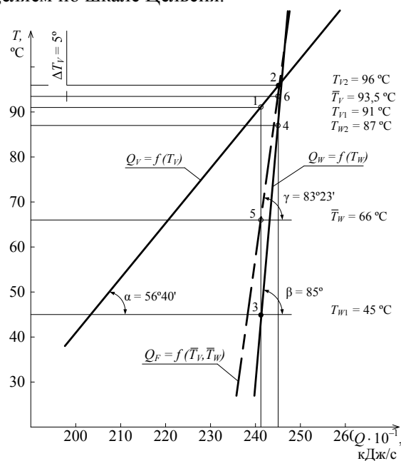
Рис. 4. Схема для решения задачи 1 по определению расхода ЖТ
