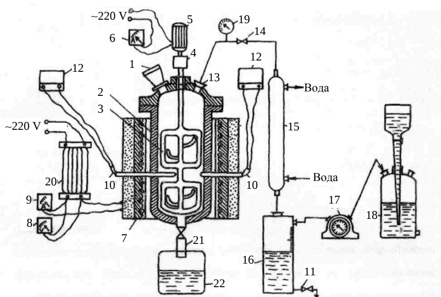
Рис. 1. Схема установки для получения термопластика из бурых углей: 1 – бункер; 2 – реактор; 3 – мешалка-ротор; 4 – редуктор; 5 – электродвигатель; 6 – амперметр, регистрирующий вязкость массы; 7 – электропечь; 8 – вольтметр и 9 – амперметр, контролирующие работу электропечи; 10 – термopара; 11 – вентиль слива жидких продуктов; 12 – потенциометр ПСР-01-03; 13, 14 – штуцер и вентиль парогазовой смеси; 15 – холодильник; 16 – приемник жидких продуктов; 17 – газосчетчик; 18 – газосборник; 19 – манометр; 20 – трансформатор; 21, 22 – штуцер и приемник термопластика
