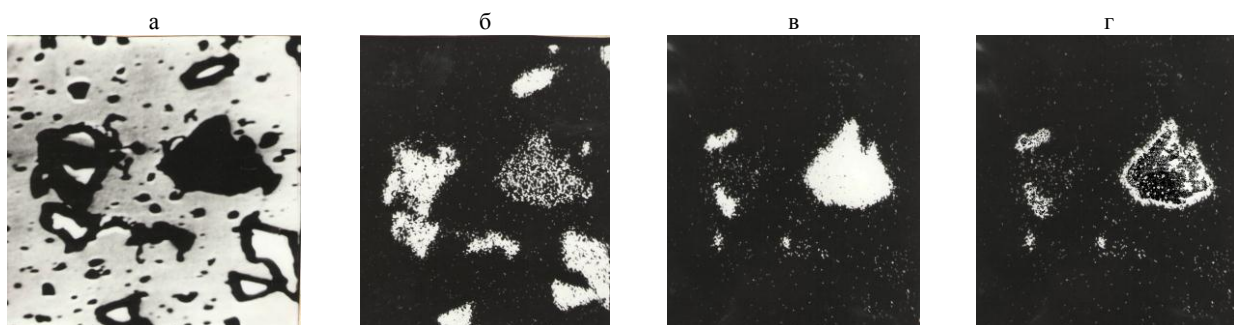
Рис. 6. Сканограмма распределения элементов в частицах порошка \text{Al}_2\text{O}_3\text{-TiO}_2 - 12\% ( \text{MoS}_2\text{-Ni} ) (агломерат): а – в поглощенных электронах; б – в характеристическом излучении алюминия; в – то же титана; г – то же молибдена ( \times 800 )
