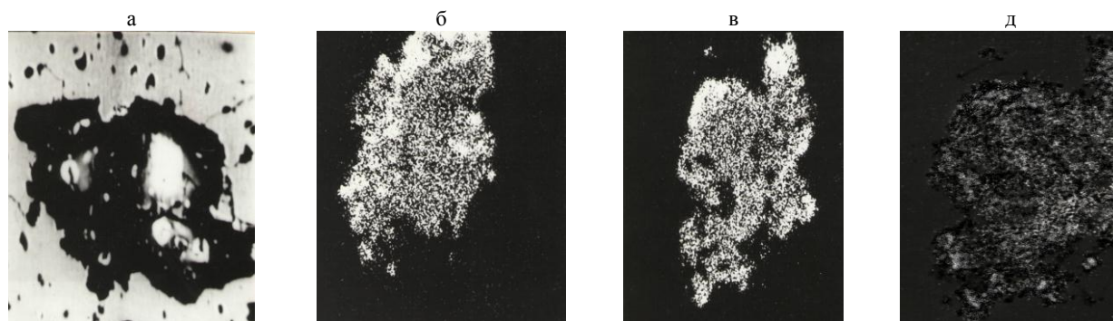
Рис. 7. Сканограмма распределения элементов в частицах порошка \text{Al}_2\text{O}_3\text{--TiO}_2\text{--}12\% (\text{MoS}_2\text{--Ni}) (CBC): а – в поглощенных электронах; б – в характеристическом излучении алюминия; в – то же титана; г – то же молибдена ( \times 800 )
