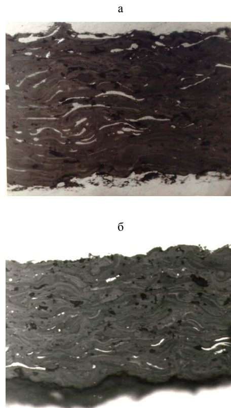
Рис. 1. Микроstructure плазменного покрытия из порошков \text{Al}_2\text{O}_3\text{--TiO}_2 - 12\% ( \text{CaF}_2\text{--Ni} ), полученных методом агломерирования мелкодисперсной шихты с последующим высокотемпературным спеканием ( \times 500 ): а – \text{Al}_2\text{O}_3\text{--TiO}_2 - 12\% ( \text{CaF}_2\text{--Ni} ); б – \text{Al}_2\text{O}_3\text{--TiO}_2 - 12\% ( \text{MoS}_2\text{--Ni} )
