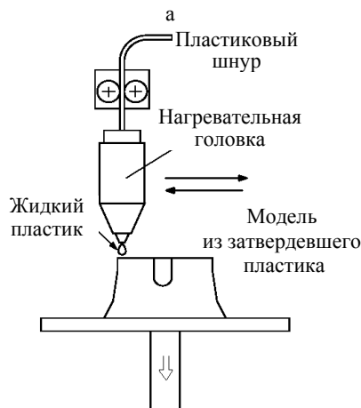
Рис. 4. Схема установки для моделирования распределением расплава (а) и образец изделия, выращенного в сборе (б)
