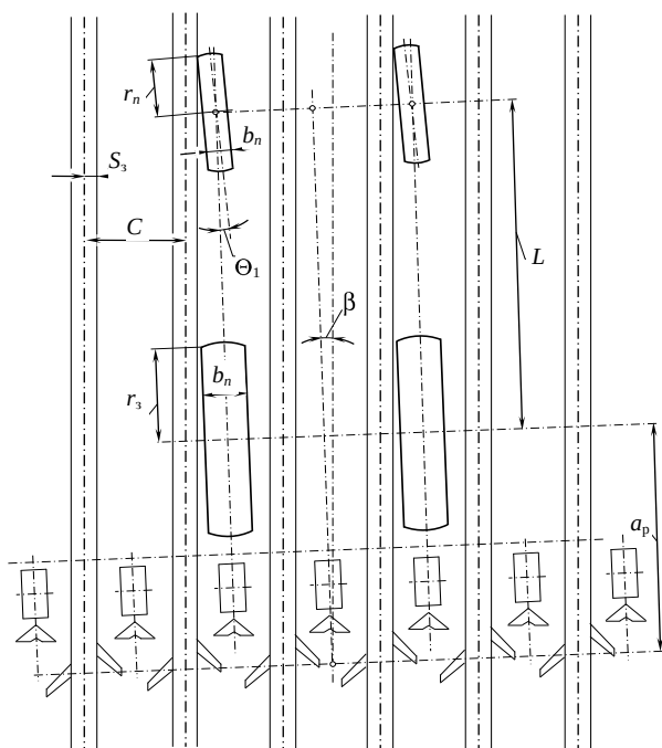
Рис. 8. Схема к определению допустимого курсового угла машинно-тракторного агрегата в междурядьях
