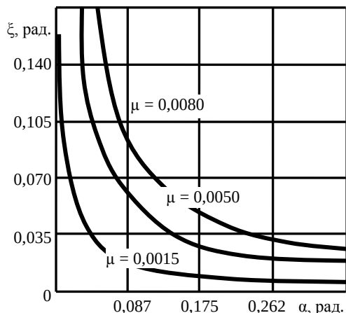
Рис. 7. Допустимые отклонения траектории агрегата от горизонтали местности в функции крутизны склона для различных допустимых уклонов траектории
