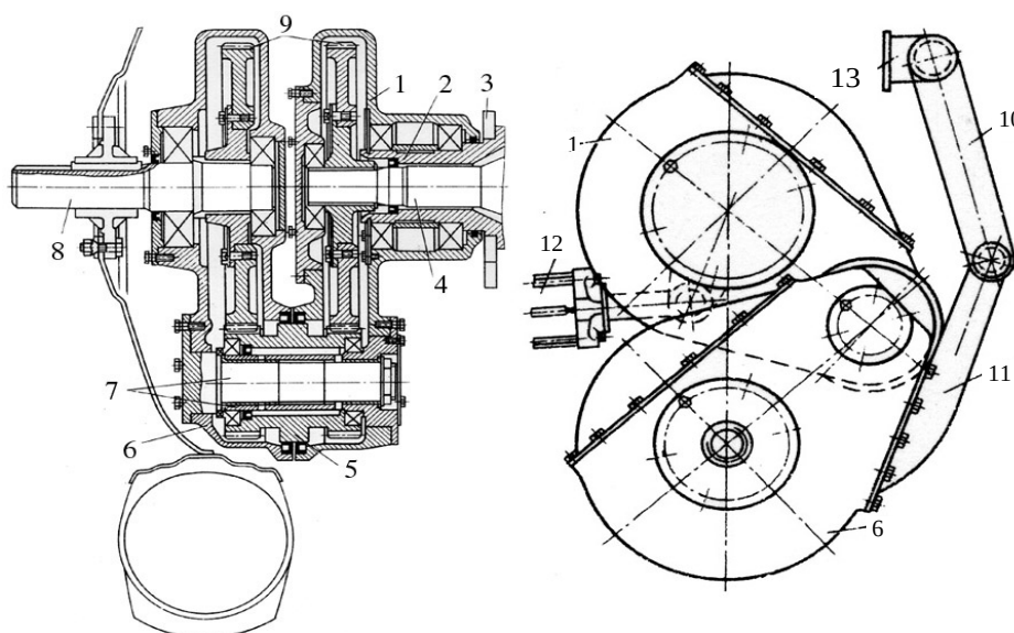
Рис. 9. Сдвоенный, раскладывающийся при стабилизации, редуктор горно-равнинной модификации трактора: 1 – первая часть редуктора, установленная на рукаве заднего моста с возможностью поворота силовым цилиндром; 2 – рукав заднего моста; 3 – фланец крепления рукава к корпусу заднего моста; 4 – ведущий вал редуктора; 5 – сдвоенная паразитная шестерня; 6 – вторая часть редуктора, поворотно сочлененная с первой и кинематически связанная с остом; 7 – цилиндрический шарнир сочленения частей редуктора; 8 – опорный вал со ступицей колеса; 9 – шестерни редуктора; 10 и 11 – тяга и рычаг кинематической связи второй части редуктора с остом; 12 – силовой цилиндр; 13 – кронштейн присоединения тяги к осту
