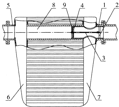
Рис. 1. Конструктивная схема охладителя наддувочного воздуха
