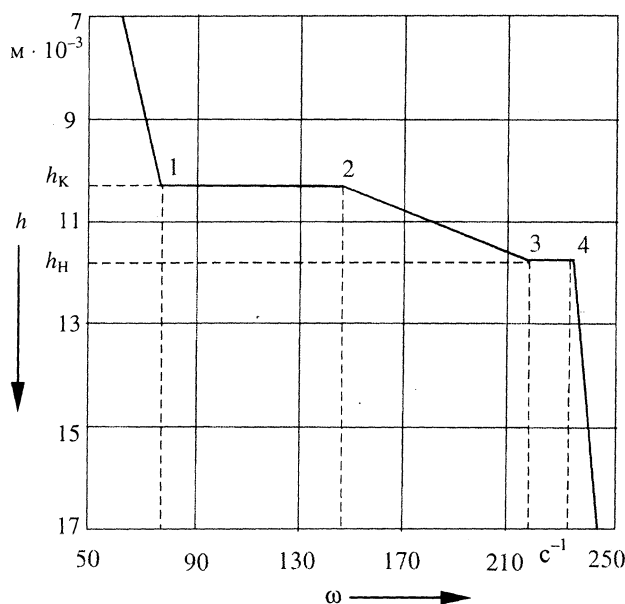
Рис. 4. Условная характеристика ТНВД
