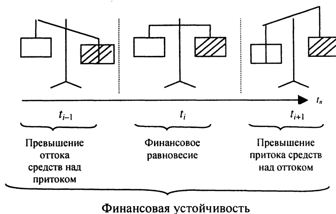
Рис. 2. Схема устойчивости при наличии финансовых разрывов: обозначения – на рис. 1
