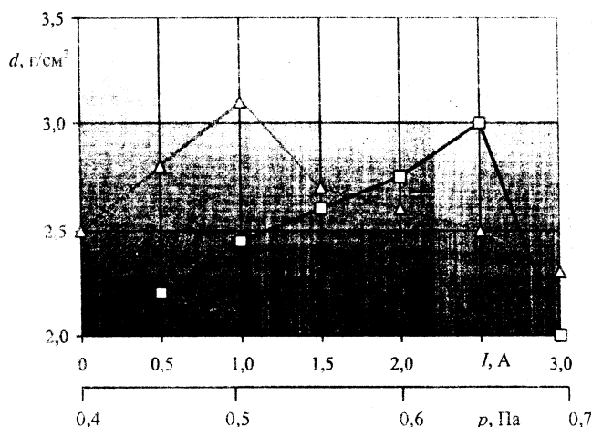
Рис. 1. Зависимость плотности углеродных покрытий от тока разряда и давления аргона: \triangle — давление Ar; \square — ток разряда
