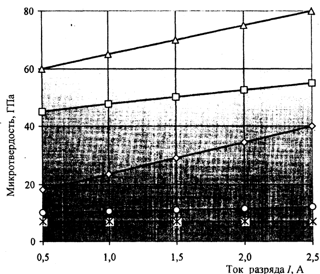
Рис. 2. Зависимость твердости углеродных покрытий от тока магнетронного разряда при различных расстояниях «мишень-подложка»: —Δ— — 150 мм, раздельный синтез; —□— — 150; —◇— — 100; —○— — 50; —*— — 30 мм
