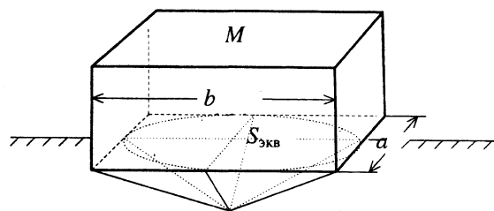
Рис. 2. Взаимодействие обрушаемого объекта и грунта
