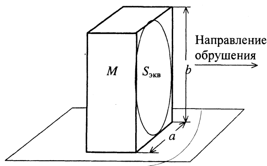
Рис. 1. Схема обрушаемого объекта с сосредоточенной массой
