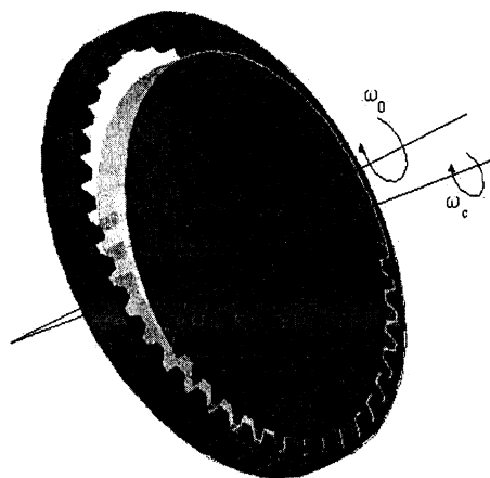
Рис. 2. Процесс формирования пространственных зубьев сателлита
