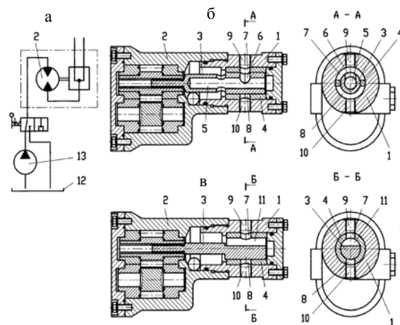
Рис. 1. Двухпоточная дозирующая система с постоянными характеристиками расхода по напорным магистралям потребителей: а – гидравлическая схема включения дозирующей системы; б – гидрораспределитель с осевым и радиальным каналами вала; в – то же с сегментным пазом вала
