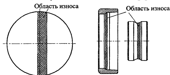
Рис. 2. Износ тел качения и колец подшипников
