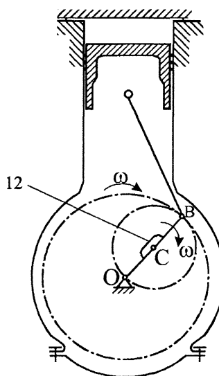
Рис. 2. Настройка установки для определения суммарных потерь мощности на трение в ЦПГ (обозначения – на рис. 1)
