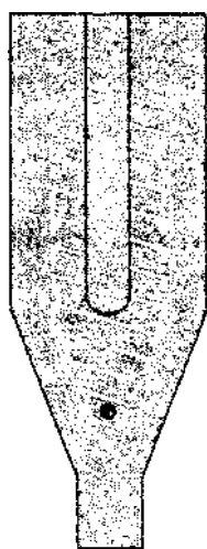
Рис. 4. Участок перехода дороги с двусторонним движением в дорогу с односторонним движением; слева - схематический план; справа - конец участка дороги с двусторонним движением, отгон две полосы
