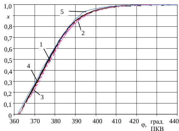
Рис. 5. Интегральная характеристика выгорания топлива при применении дизельного, смесевых топлив и метилового эфира: n = 2200 \text{ мин}^{-1} ; 1 – ДТ; 2 – 5 % МЭЖК; 3 – 30 % МЭЖК; 4 – 50 % МЭЖК; 5 – 100 % МЭЖК
