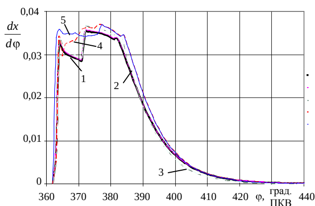
Рис. 4. Расчетная дифференциальная характеристика выгорания топлива при применении дизельного, смесевых топлив и метилового эфира: n = 2200 \text{ мин}^{-1} ; 1 – ДТ; 2 – 5 % МЭЖК; 3 – 30 % МЭЖК; 4 – 50 % МЭЖК; 5 – 100 % МЭЖК
