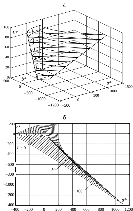
Рис. 7. Цветовое тело самосветящихся объектов: а – в колориметрической системе L^*a^*b^* при освещении/наблюдении D65/1964 и границы монохроматических стимулов; б – при варьировании L = 0 - 100 с шагом 10
