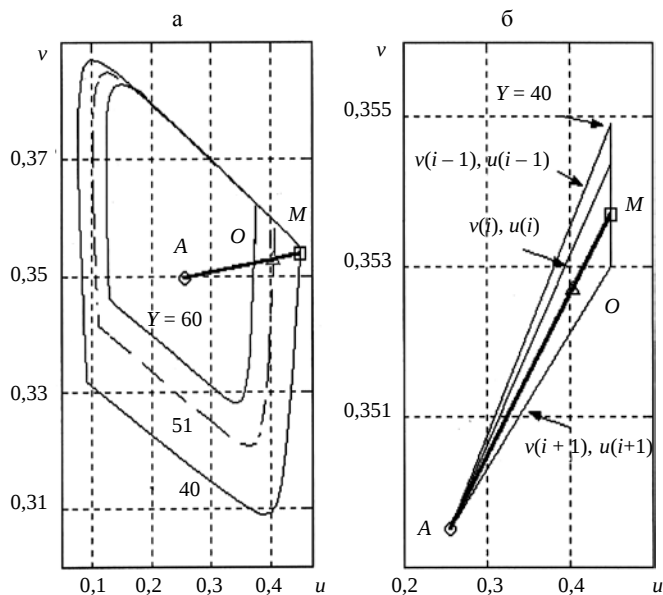
Рис. 3. а – (u-v) -график с границами оптимальных цветовых стимулов при Y = 40, 51 и 60 ; б – участок графика, используемый для определения чистоты цвета; A – координаты цветности источника освещения ( x = 0,4476 ; y = 0,4075 ); O – координаты цветности задаваемого покрытия ( x = 0,6100 , y = 0,3550 ); M – координаты цветности точки максимальной чистоты цвета при регламентированном Y = 40 ; A - v(i-1), u(i-1) - v(i), u(i) и A - v(i),
