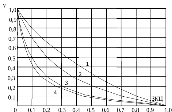
Рис. 9. Зональные (яркостные) коэффициенты цветопередачи при варьировании Y = 0-100 с шагом 10 для некоторых источников стандартного излучения: 1 – D65/1964; 2, 4 – F/1931 (люминесцентные лампы; 2 – Daylight, коррелированная цветовая температура 3000 K; 4 – Standard Warm White, коррелированная цветовая температура 3000 K [4]); 3 – A/1931
