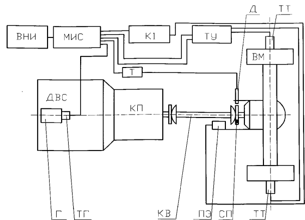
Рис. 1. Принципиальная схема подключения датчиков и измерительных модулей: МИС – многоканальная измерительная система «М3 INTEGRA 1»; Т – тахометр ТАС-100; К1 – преобразователь одноканальной телеметрической системы; ТУ – тензоусилитель KWS-3073; Д – оптический датчик частоты вращения; ТТ – токосъемники SK-6; Г – генератор; ТГ – тахогенератор MEZ K4A2; ДВС – двигатель внутреннего сгорания; КП – коробка передач; КВ – карданный вал; ПЭ – приемный элемент телеметрической системы К1; СП – пластина со светоотражающей поверхностью; ВМ – ведущий мост; ВНИ – внешний носитель информации
