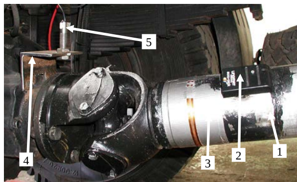
Рис. 3. Монтаж датчика частоты вращения и телеметрической системы на автомобиле МАЗ-544008: 1 – карданный вал; 2 – статор К1-Р2; 3 – силовая обмотка; 4 – кронштейн крепления датчика частоты вращения; 5 – оптический датчик частоты вращения
