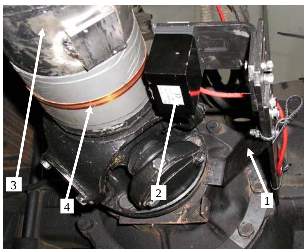
Рис. 2. Монтаж телеметрической системы на карданном валу автомобиля МАЗ-544008: 1 – кронштейн крепления приемного элемента; 2 – приемный элемент К1-С4; 3 – карданный вал; 4 – силовая обмотка
