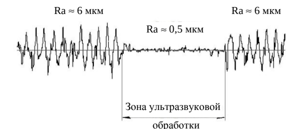
Рис. 3. Профилограмма поверхности чугуна СЧ20 – исходная и после УЗППД (параметры УЗППД: частота УЗ колебаний – 18 кГц; амплитуда колебаний – 20–25 мкм; усилие статического прижима – 45 кг; поперечная подача деформирующего элемента – 0,6 мм/об; продольная скорость перемещения деформирующего элемента – 2,6 м/мин)
